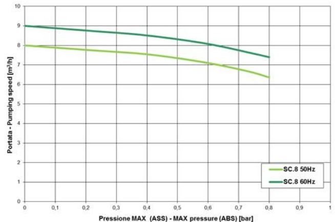
COMPRESSORE / COMPRESSOR
